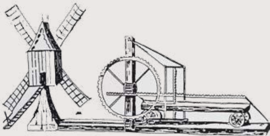
Tekening van de krukas bij het octrooi uit 1593
