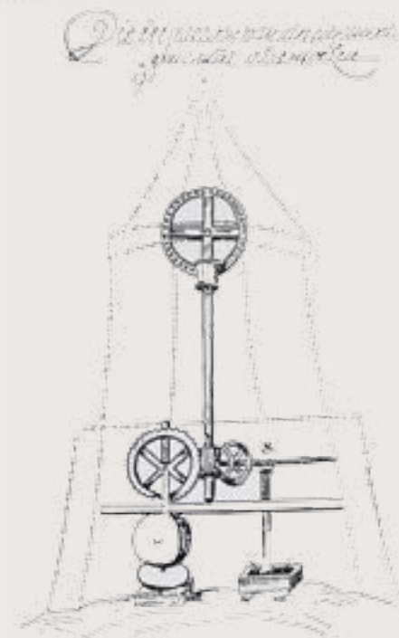
Tekening met kantstenen uit het octrooi van 1597
