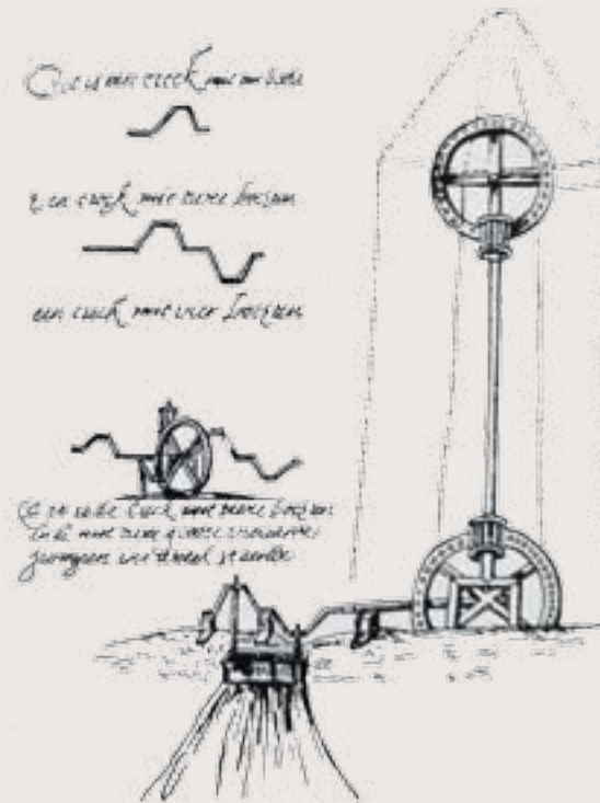
Tekening van de krukas met 1, 2 en 4 bochten bij het octrooi uit 1597
